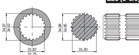
Z21 (1"3/8)
